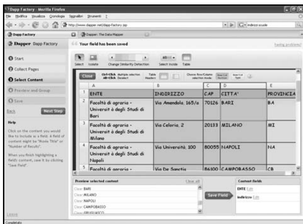
Figura 1.2: Estrazione degli indirizzi.
